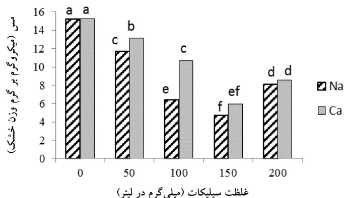
شکل ۸. اثرهای متقابل منبع و غلظت سیلیکات در محیط کشت خاک بر میزان عنصر مس برگ داوودی. حروف غیرمشابه نشان‌دهنده وجود اختلاف معنی‌دار در آزمون دانکن در سطح ۱٪ است.
