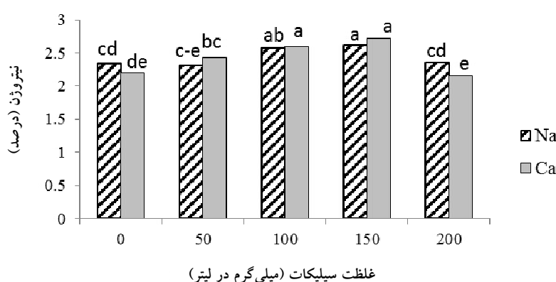
شکل ۲. اثرهای متقابل منبع و غلظت سیلیس در محیط کشت خاک بر میزان عنصر نیتروژن برگ داوودی. حروف غیرمشابه نشان‌دهنده وجود اختلاف معنی‌دار در آزمون دانکن در سطح ۱٪ است.
