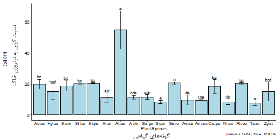
شکل ۴. مقایسه میانگین نسبت کربن به نیتروژن خاک در رویشگاه‌های مورد مطالعه (داده‌های اصلی). ستون‌های دارای حداقل یک حرف مشترک، تفاوت معنی‌داری در سطح احتمال ۵ درصد ندارند.
