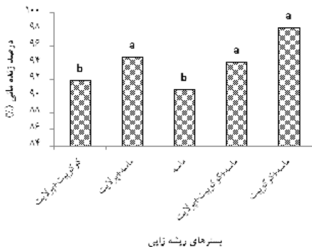
شکل ۱. اثر تیمارهای مختلف بر درصد زنده ماندن قلمه‌های ریشه‌دار شده گیاه شیشه‌شور پس از انتقال به گلدان. میانگین‌هایی که دارای حداقل یک حرف مشترک هستند از لحاظ آماری در سطح احتمال ۵٪ فاقد اختلاف معنی‌دار می‌باشند.
