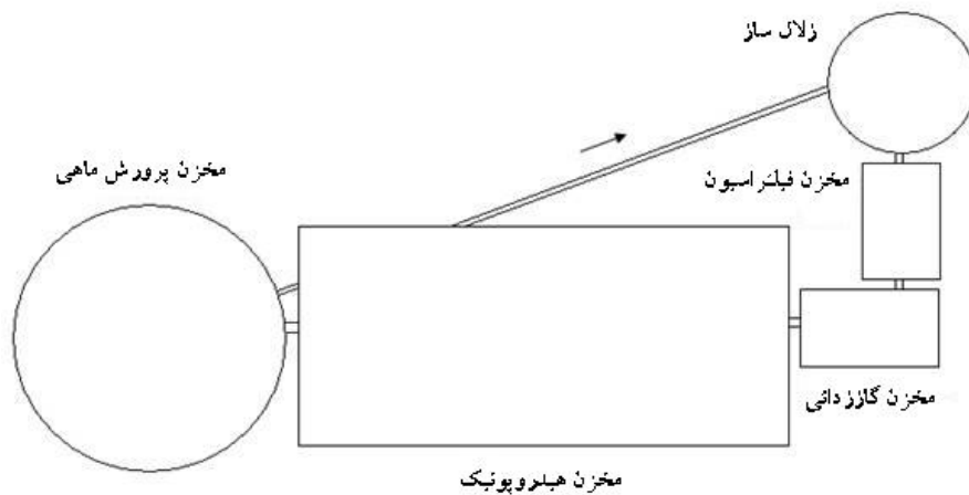
شکل ۱. طرح سیستم آکواپونیک در دانشگاه ولیعصر (عج) رفسنجان
