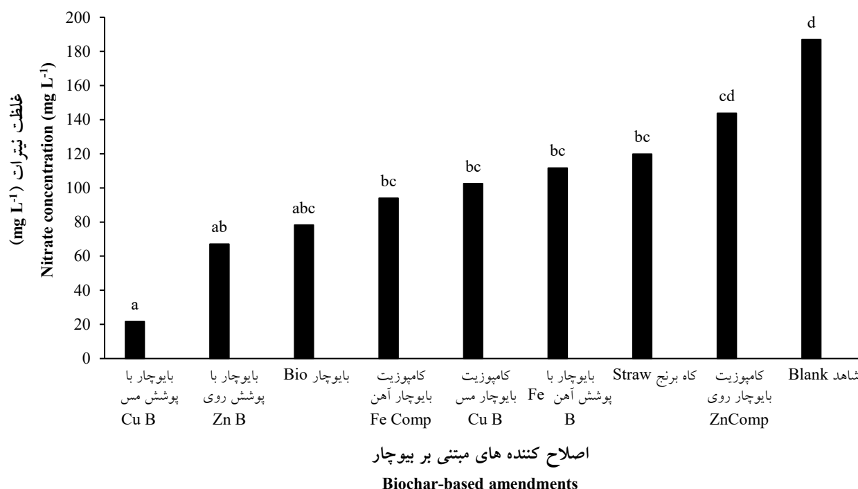
شکل ۲. مقایسه تأثیر اصلاح کننده های مبتنی بر بیوچار بر غلظت نترات در زه آب حاصل از آبشویی پیوسته
