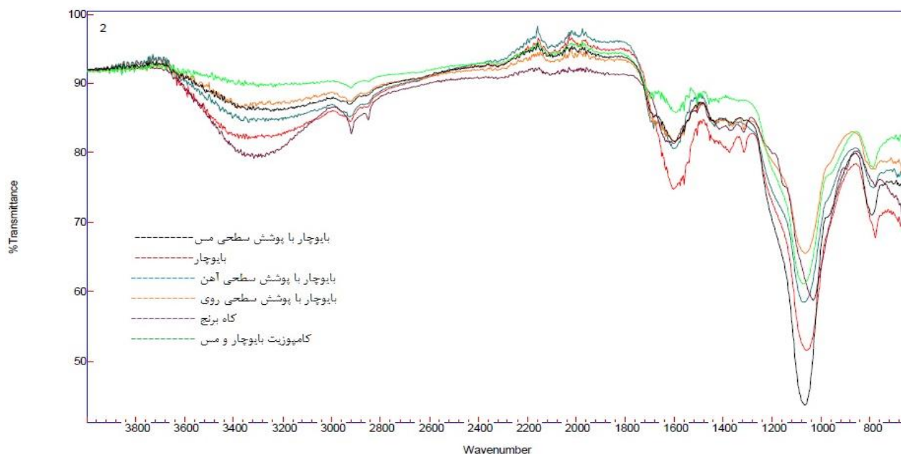
شکل ۱. طیف مادون قرمز بیوچار و بیوچارهای با پوشش سطحی فلزی مورد بررسی
