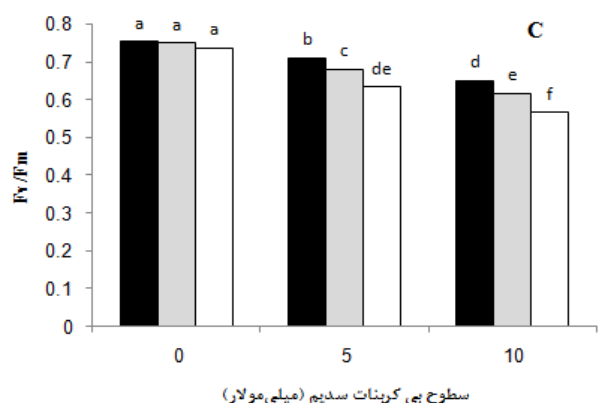
شکل ۲. اثر متقابل سطوح بی‌کربنات سدیم و منابع آهن بر کلروفیل a (A)، کلروفیل b (B) و F_v/F_m (C) در گیاه کاهو. حروف متفاوت در بالای ستون‌ها نشان‌دهنده اختلاف معنی‌دار بین تیمارها در سطح ۵٪ آزمون دانکن است.
